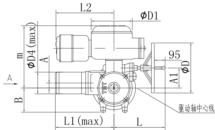
QBR3Ex. IN~QBR5Ex. IN系列外形尺寸
